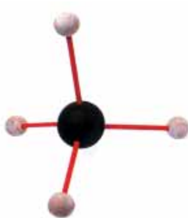
Struktura e gazit metan: Përreth atomit të karbonit në mes, janë lidhur katër atome të njëjtë hidrogjeni.
