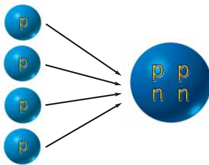
Bërthama hidrogjeni me nga një proton
