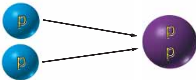
Bërthama e "di-protonit" me dy protone
