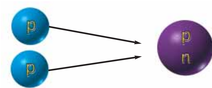
Bërthama hidrogjeni me nga një proton
